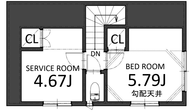
3F : 23.07 m 2
