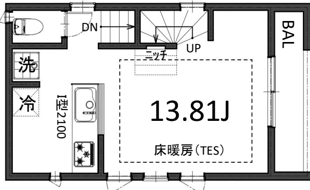
2F : 29.56 m 2
